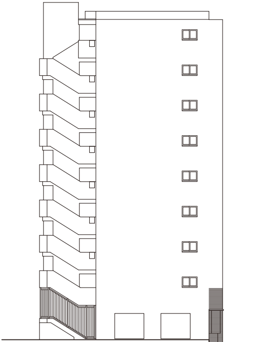
東側立面图
