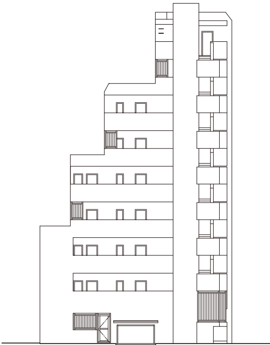
南側立面图
