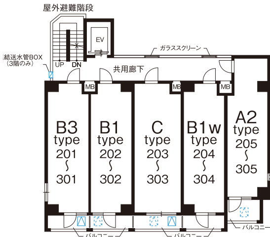
2~3階平面図
