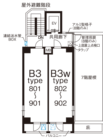
8~9階平面図
