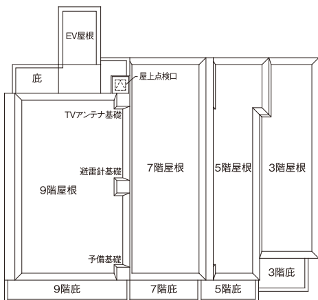
屋上平面図
