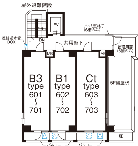
6~7階平面図
