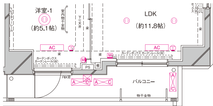
7階部分図
